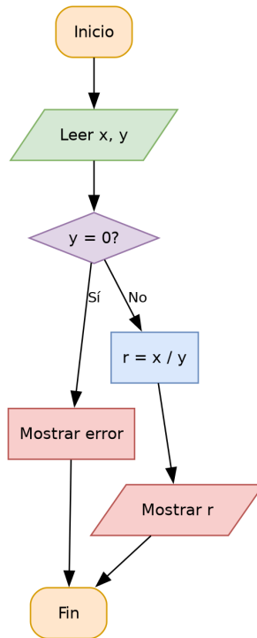
Figura 3.14: Diagrama de flujo de Division (P1).
