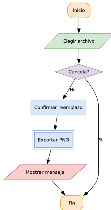
Figura 3.26: Diagrama de flujo de EditorFrame (P1).
