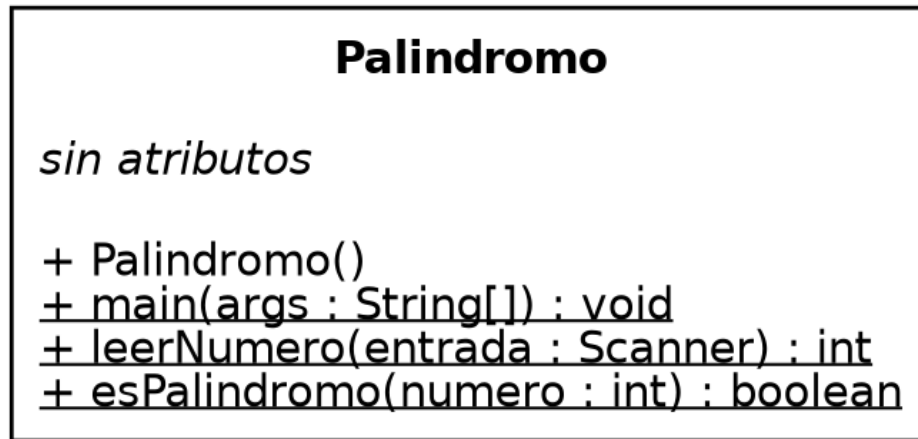
Figura 3.33: Diagrama UML de Palindromo (P3).
