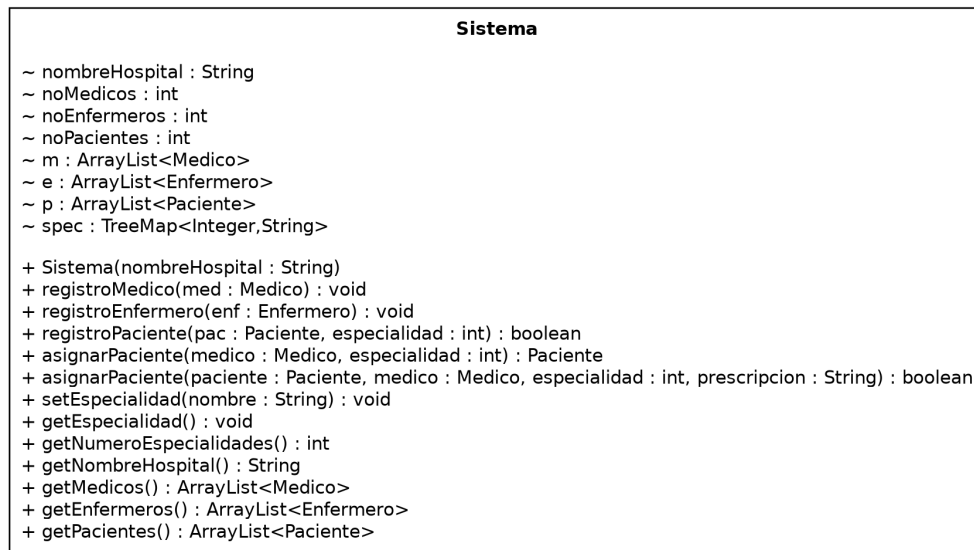
Figura 3.53: Diagrama UML de Sistema (Proyecto).
