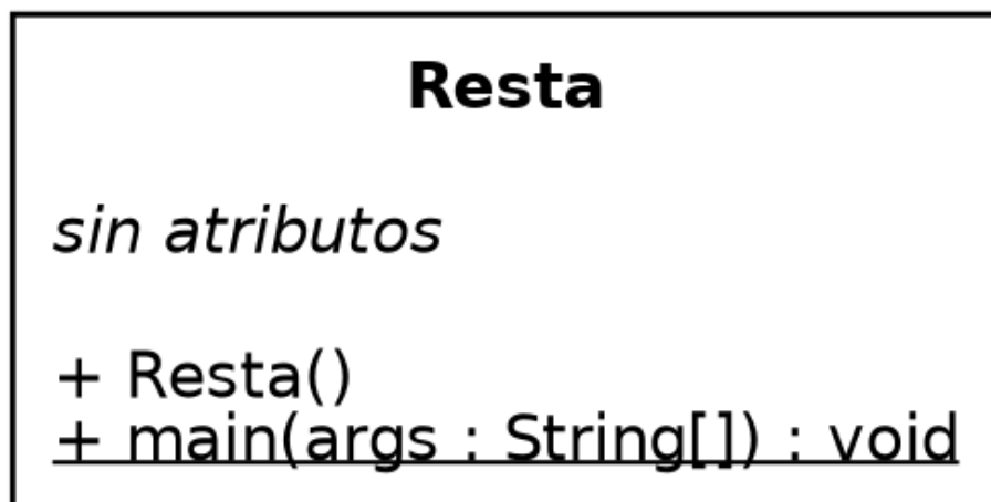
Figura 3.9: Diagrama UML de Resta (P1).
